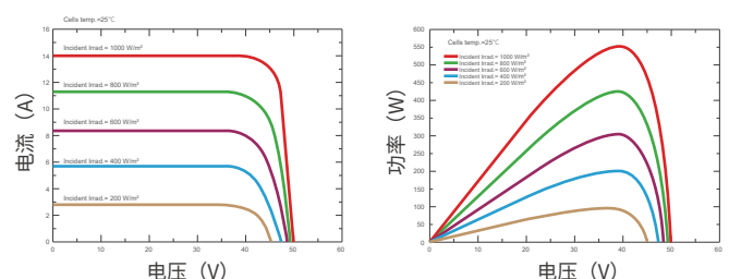
电流电压及功率电压曲线 (SKT555M10)
