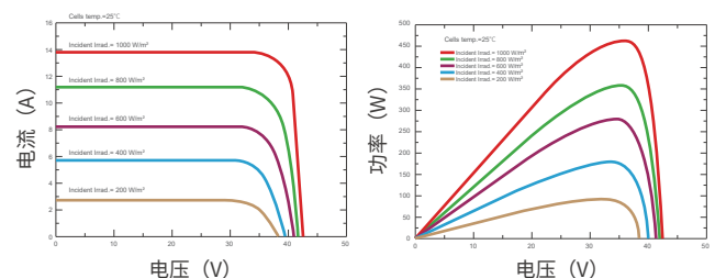
电流电压及功率电压曲线 (SKT460M10)
